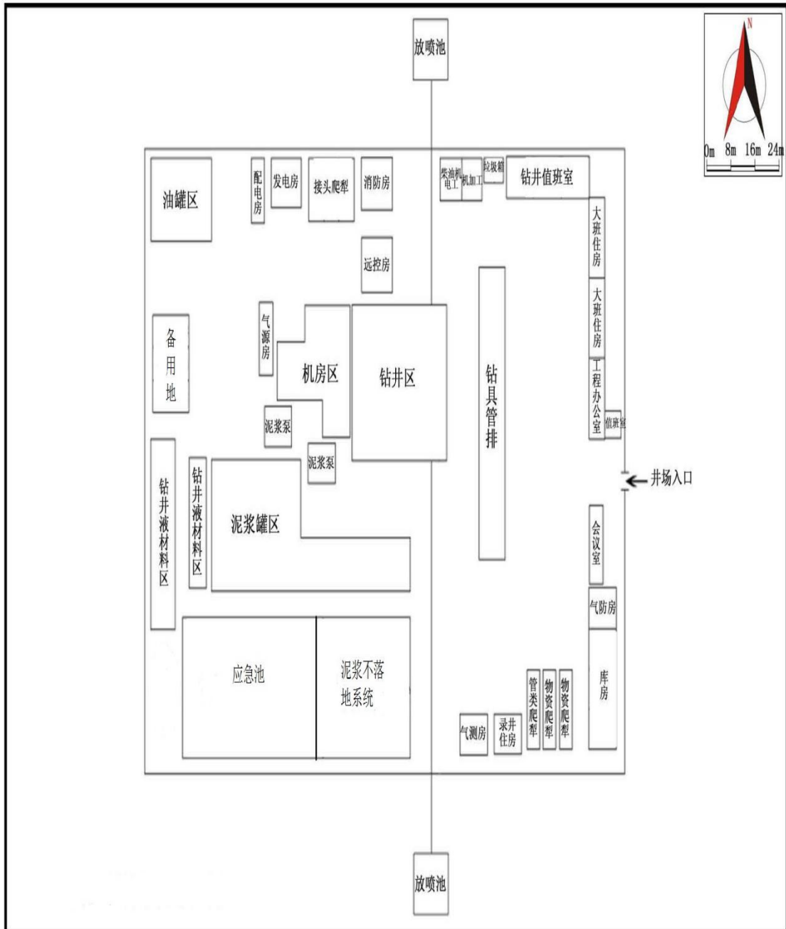
图 4-3 钻井期井场平面布置示
