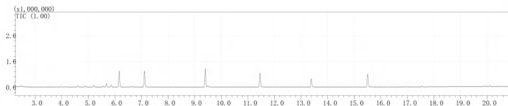
图 9-2 样品的 VOCs 的总离子流图 (TIC) (含内标、替代物及柱流失硅氧峰)
