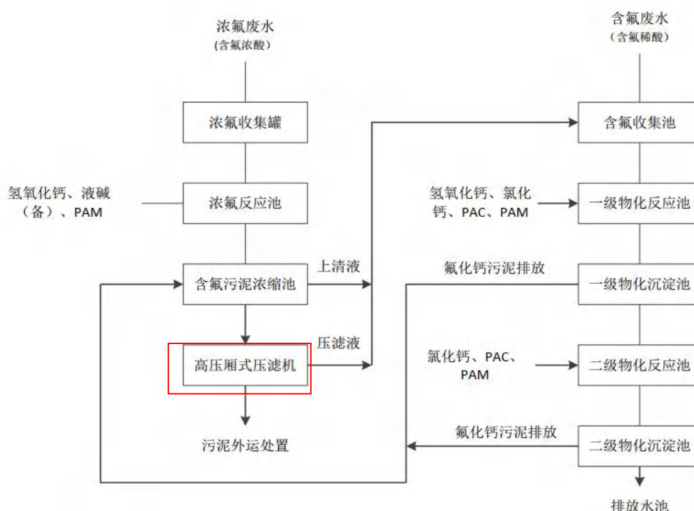
图 7-5 含氟废水处理系统工艺流程示意图
