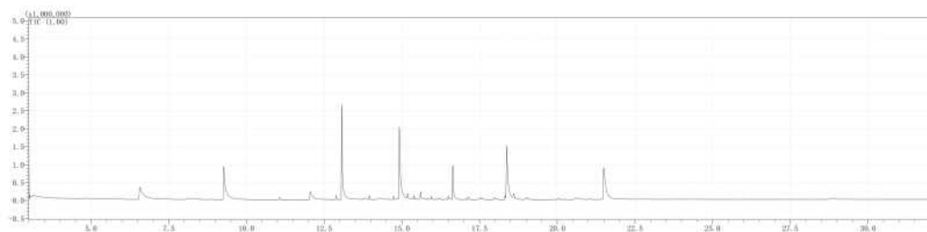
图 9-4 空白的 SVOCs 总离子流图 (TIC) (含内标、替代物及柱流失硅氧峰)
