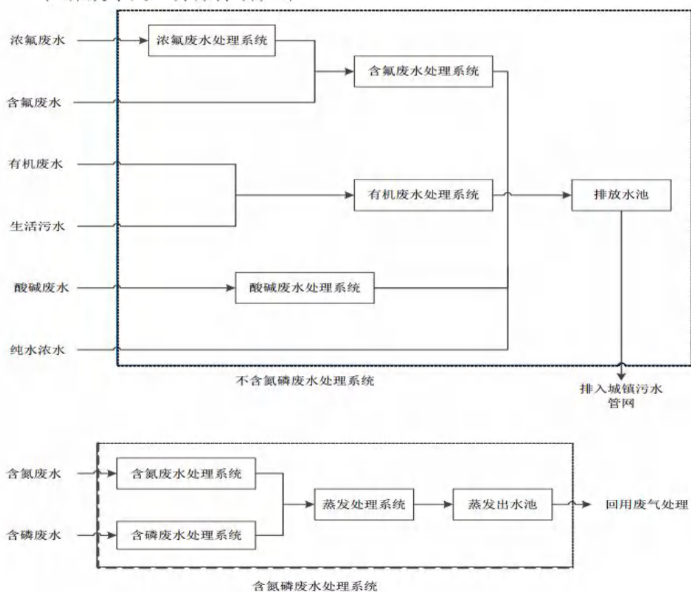
图 7-4 废水处理流向图
