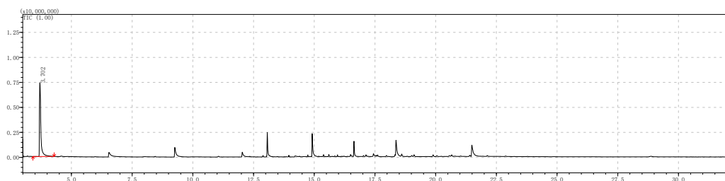
图 9-6 样品的 SVOCs 的总离子流图 (TIC) (含内标、替代物及柱流失硅氧峰)
