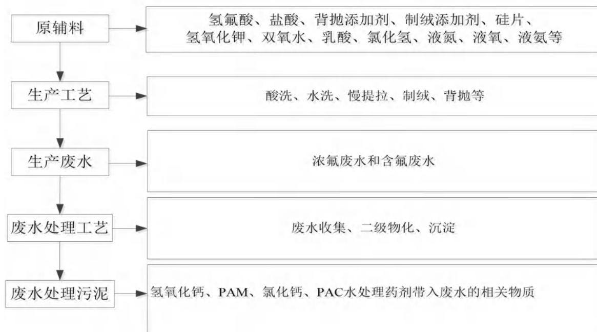
图 7-7 污泥污染物迁移路线图
