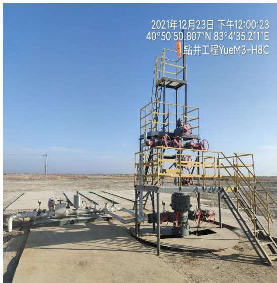
采油树
