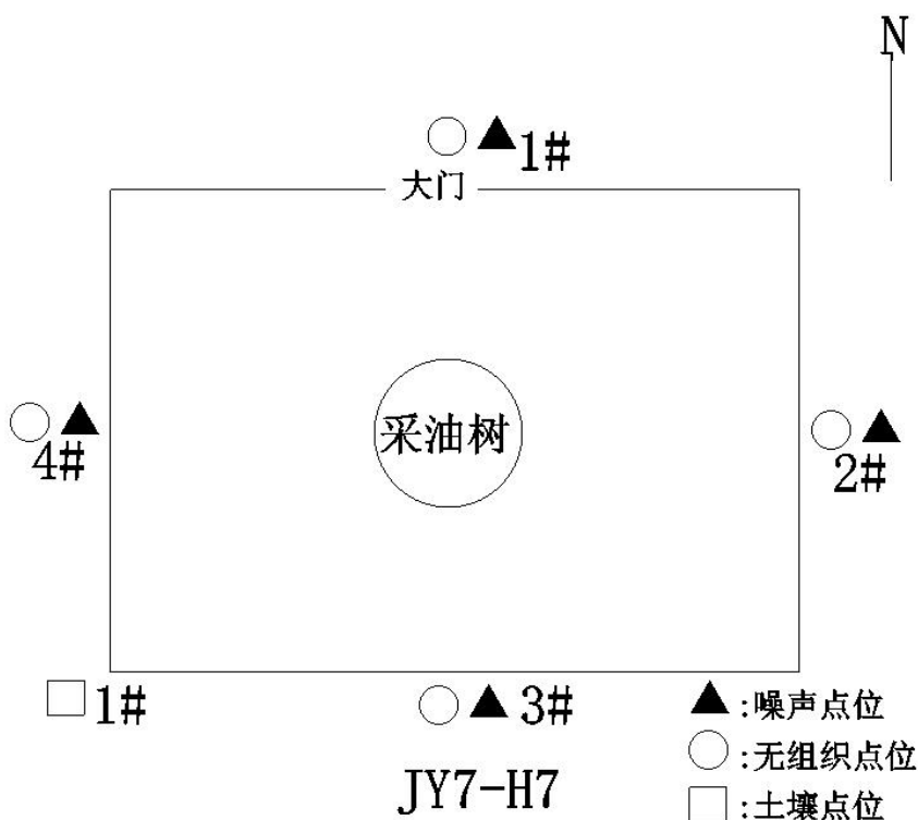
图 8-1 JY7-H7 井监测点位图
