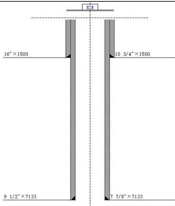
图 4-4 实际井身结构图
