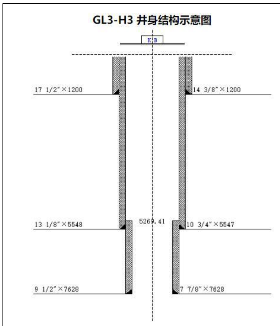
图 4-5 井身结构图
