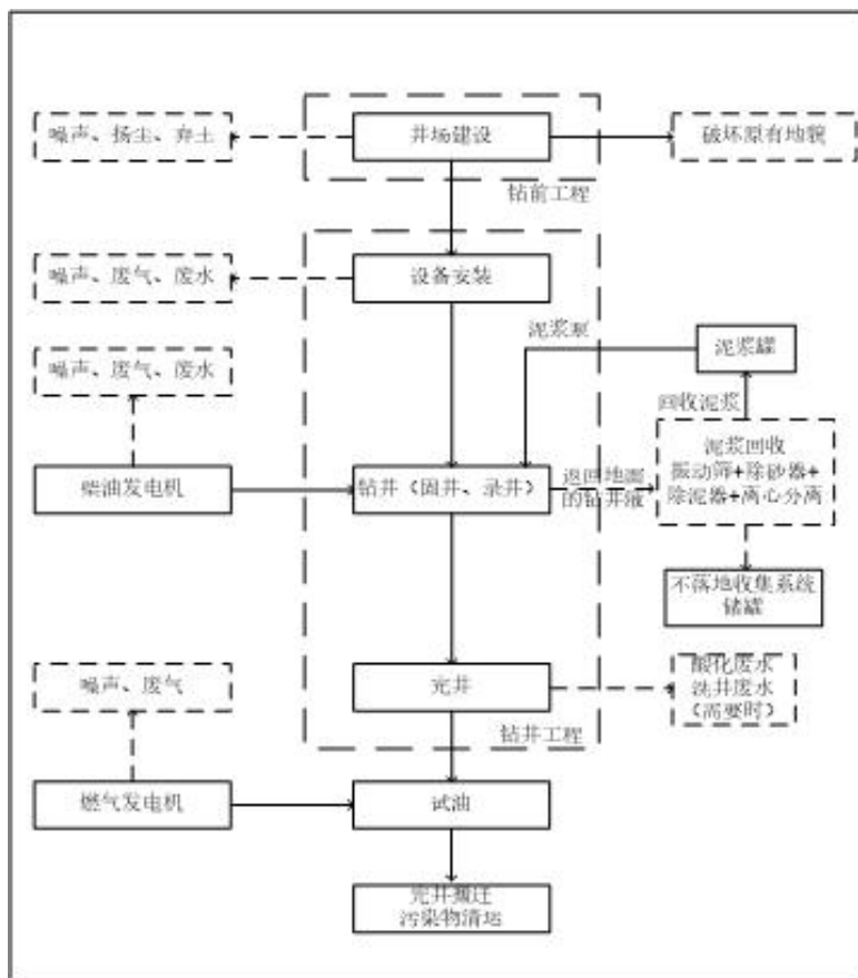
图 4-5 工艺过程示意图
