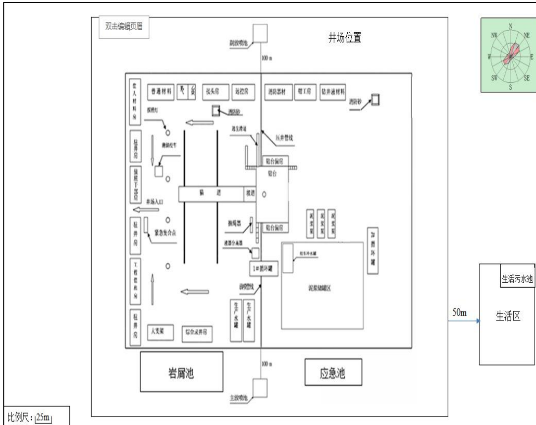
图 4-3 钻井期井场平面布置示意图
