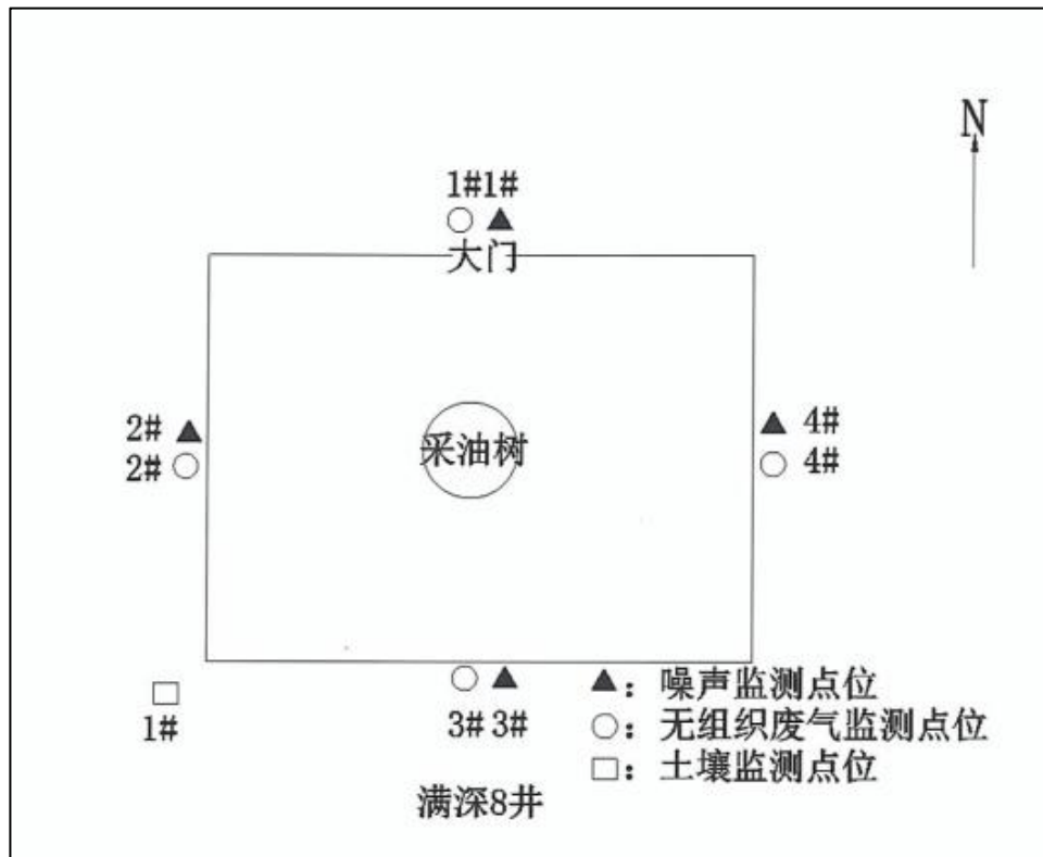
图 8-1 满深 8 井监测点位图
