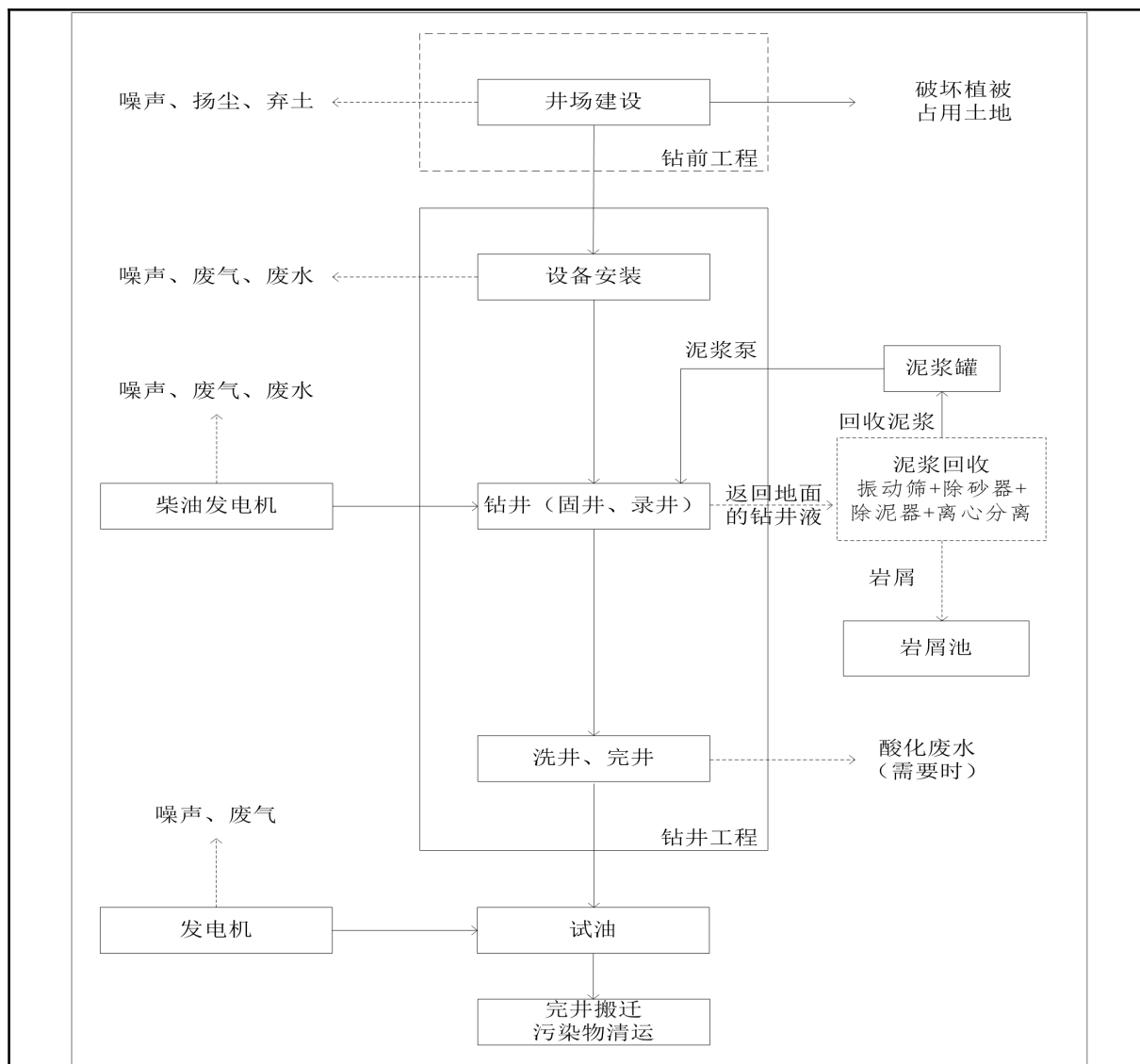
图 4-5 工艺流程示意图
