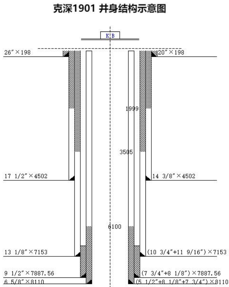
图 4-4 实际井身结构图
